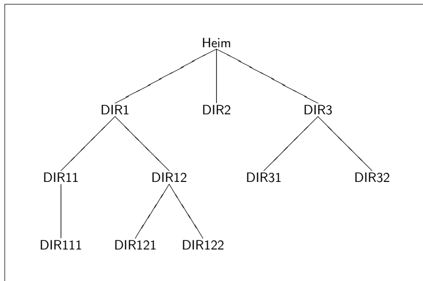
Abbildung 1: Die Verzeichnisstruktur
